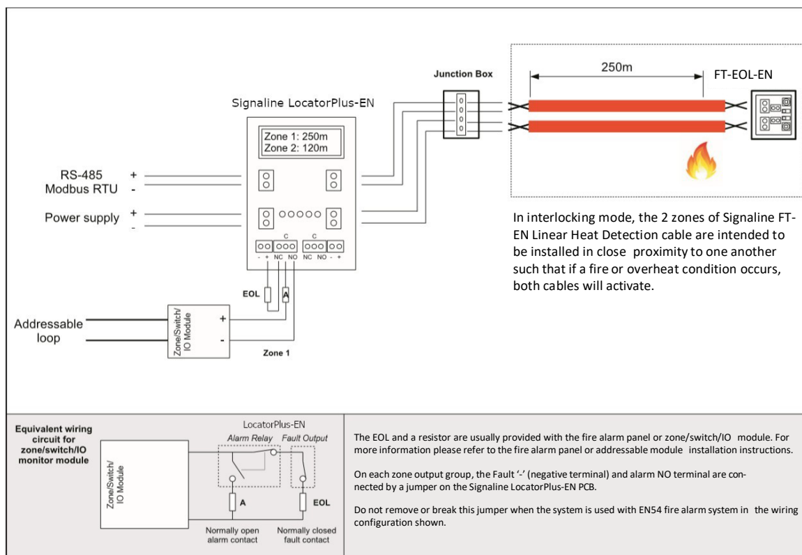
Rys. 4. Typowe podłączenie w trybie zależnym
