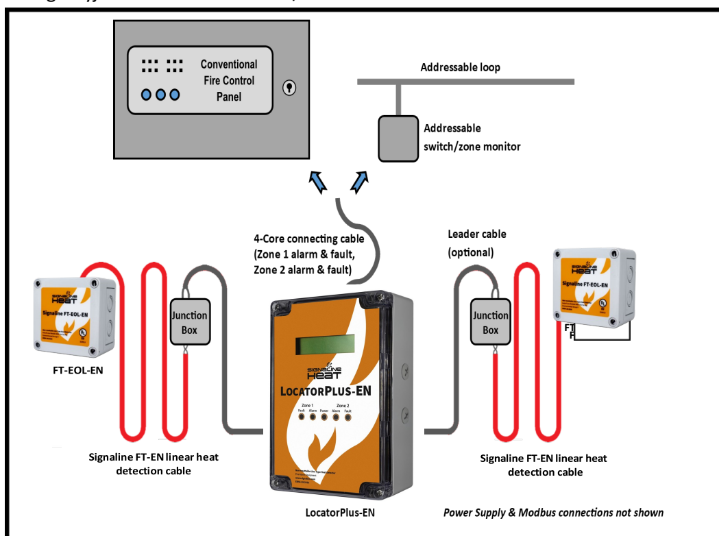
Rys 1. Typowa konfiguracja systemu
