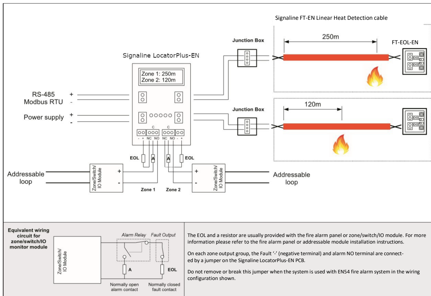
Rys. 3. Typowy schemat dla trybu pracy niezależnego
