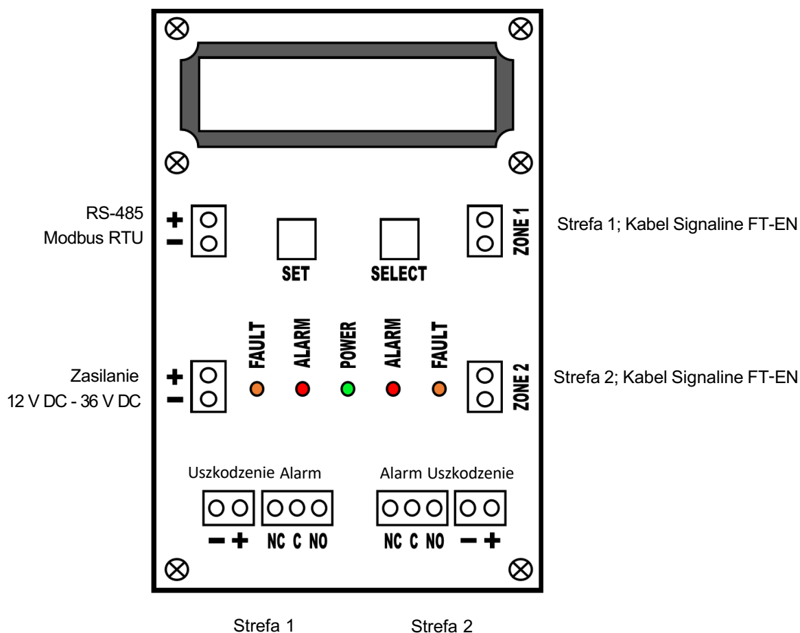
Rys 2. Podłączanie Lokalizatora Signaline LocatorPlus-EN
